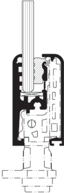
Glasdichtung waagrecht
