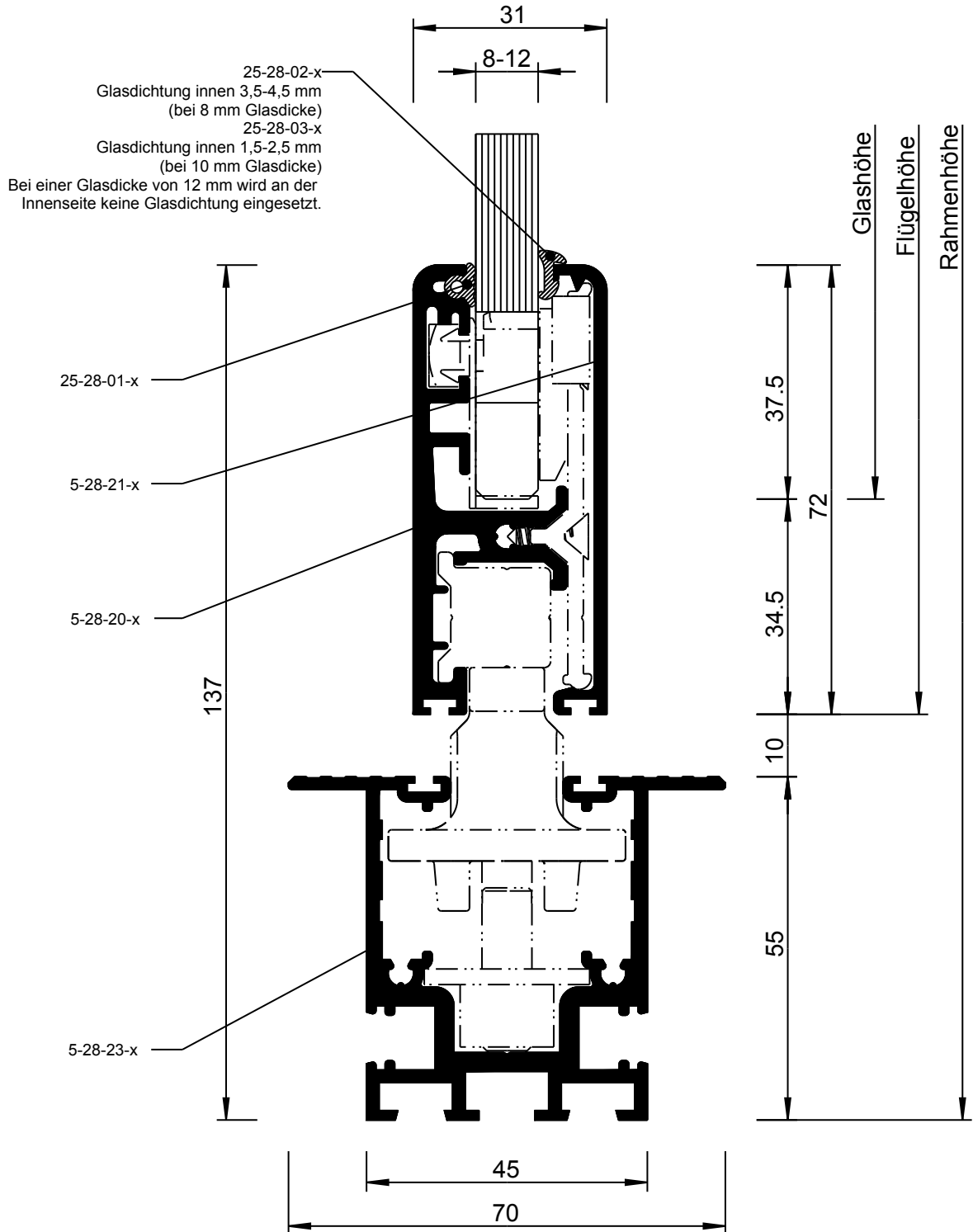
Detail 25 XXL-2-4
