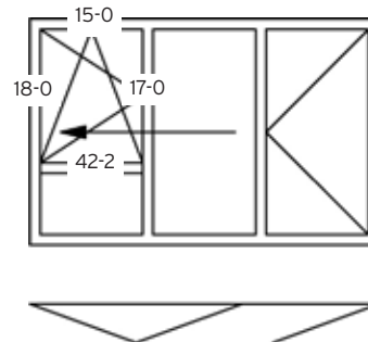
Faltwand mit Dreh-/Kippflügel im Faltflügel oberhalb Querkämpfer
