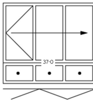
Faltwand auf Brüstung
