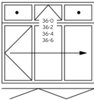
Faltwand mit Oberlicht
