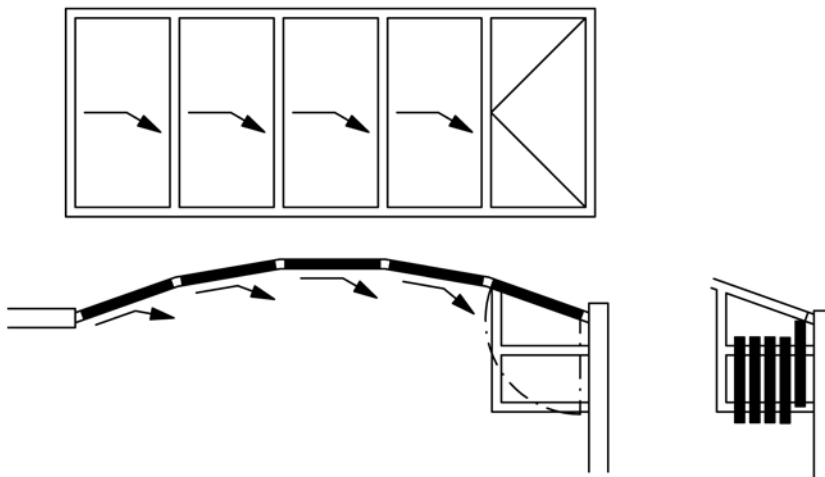
segmentierter Grundriss
