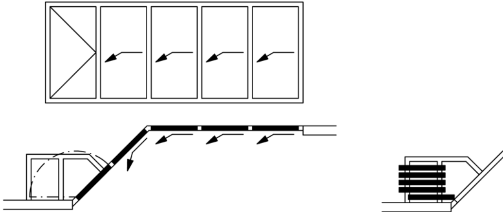
Grundriss mit einer Abwicklung
