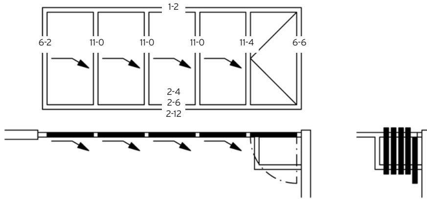
gerader Grundriss
