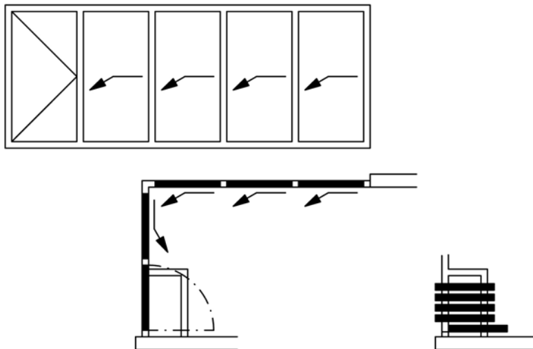
Grundriss mit 90° Ecke
