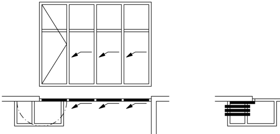
HSW mit Sprosse
