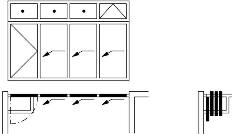
HSW mit Oberlicht
